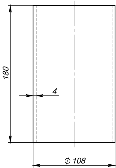
Поз.4 (Труба)
