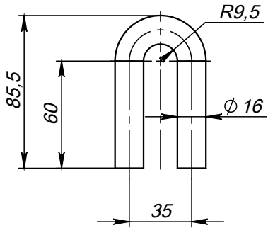
Поз.4 (Труба)
