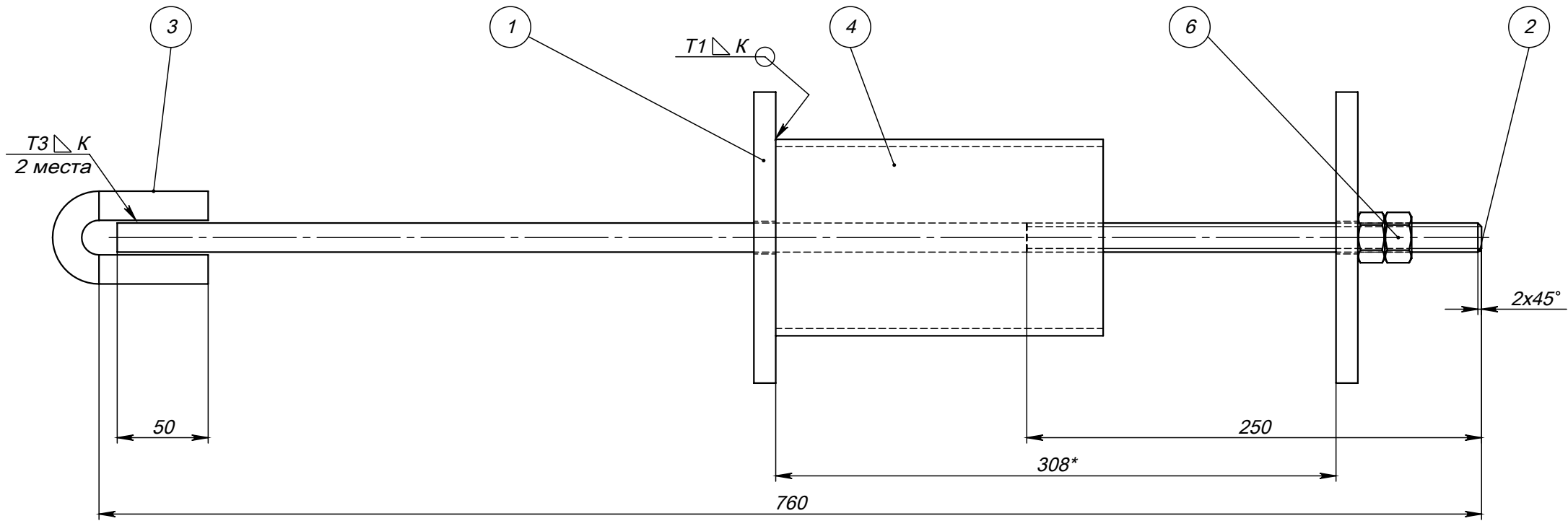
Поз.3 (Ушко)
